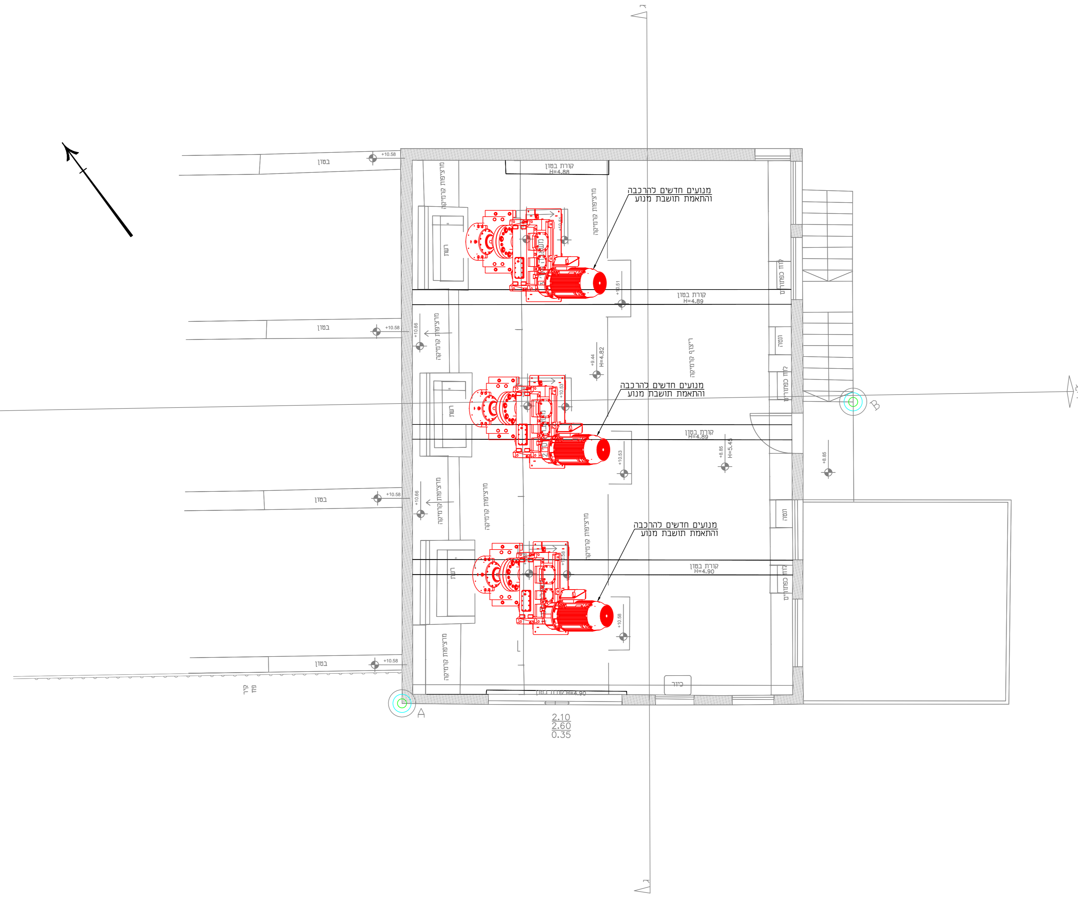
מבט על-קומת ראשונה קו"מ: 1:50
