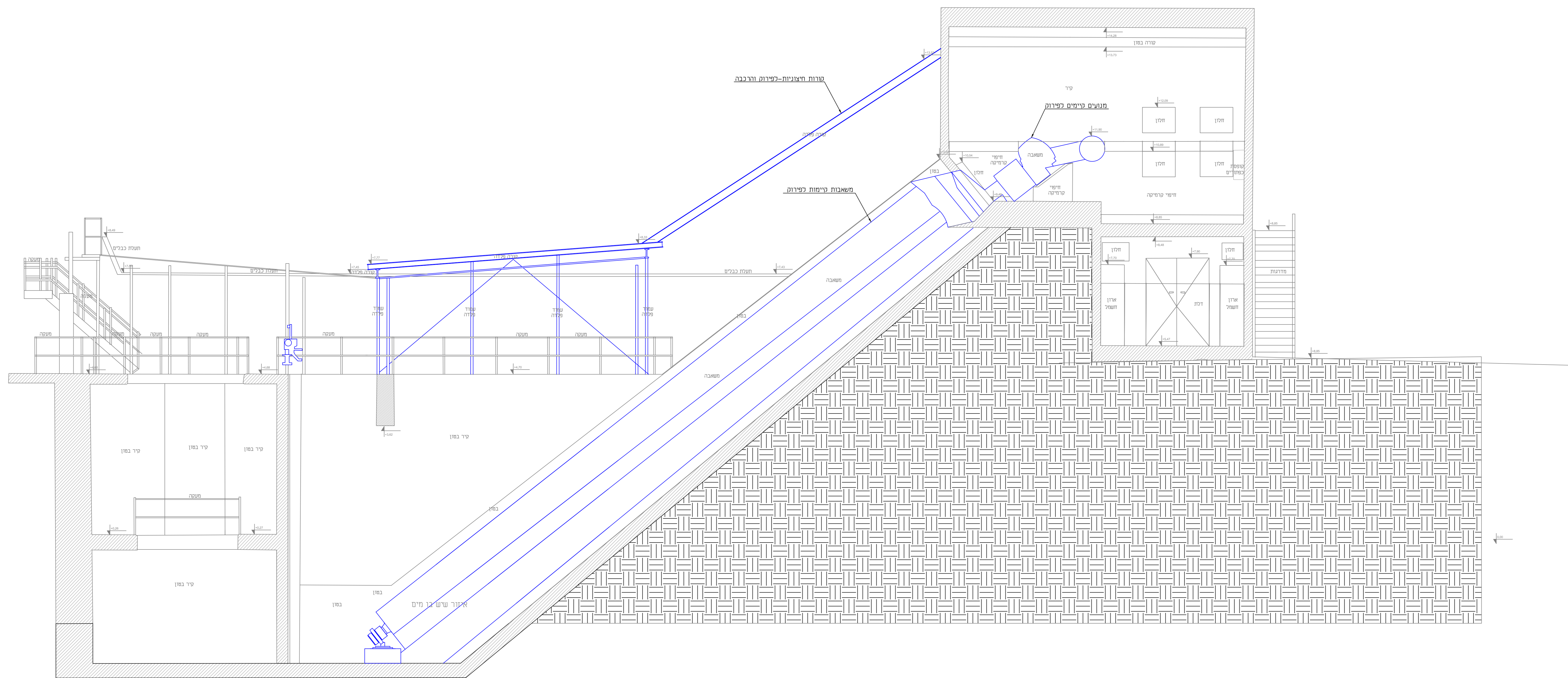
חתך א-א קו"מ: 1:50
