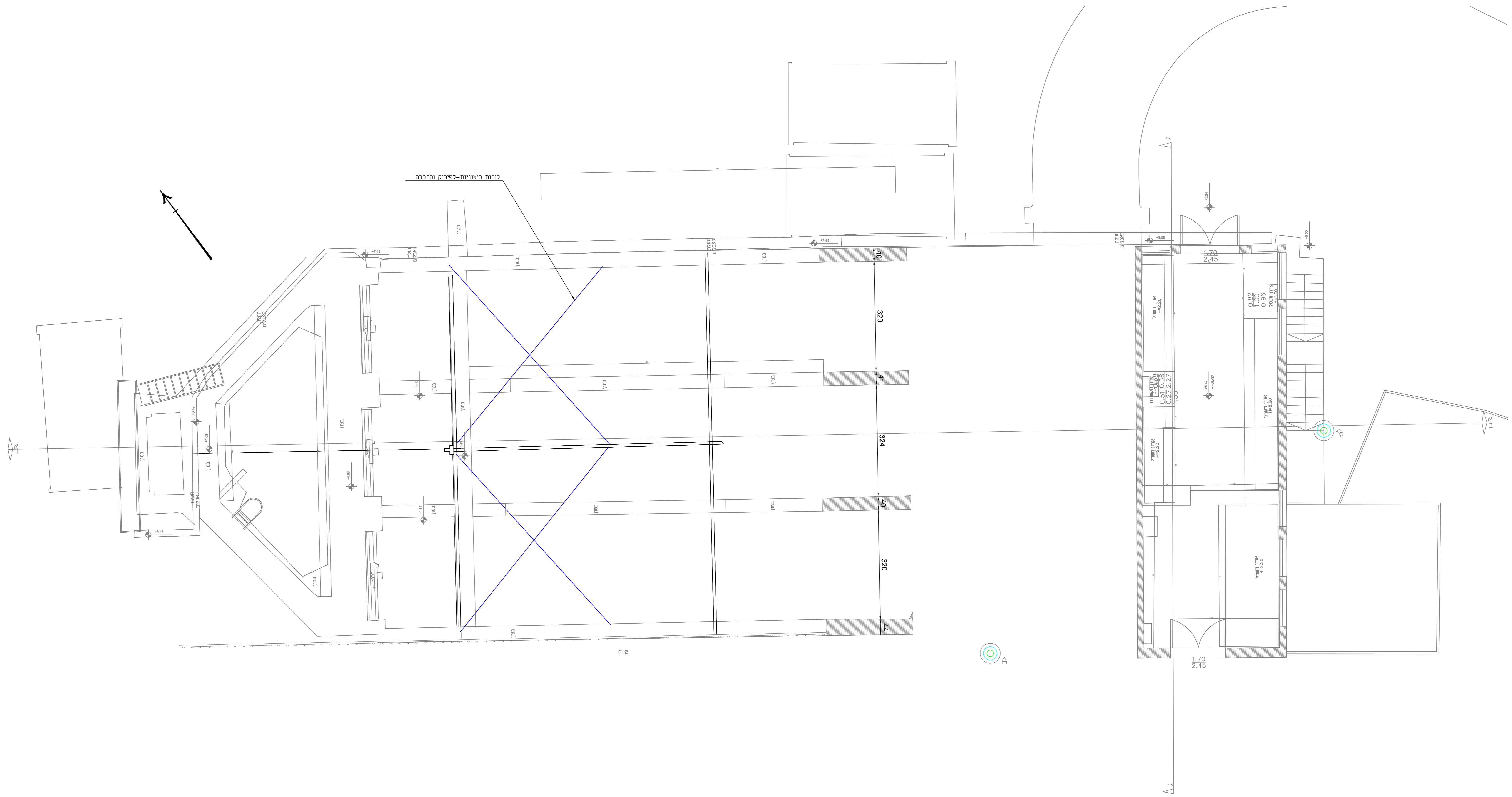
מבט על- קומת קרקע קני"מ: 1:50
